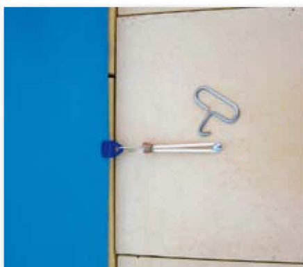
Kit antisoulèvement par pince sur toile (EA 4436)
